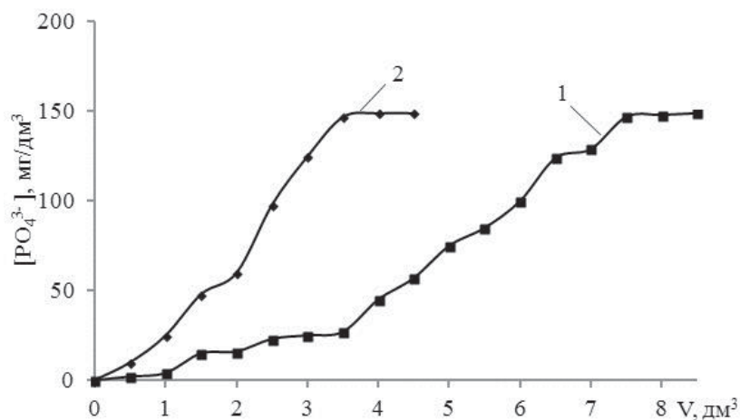
Рис. 2. Вихідні криві сорбції фосфатів на аніонітах АВ-17-8 (1) та Dowex Marathon (2) ( V_i = 10 см 3 ) в Cl - формі при фільтруванні розчинів Na 2 HPO 4 з концентрацією 170 мг/дм 3 .
