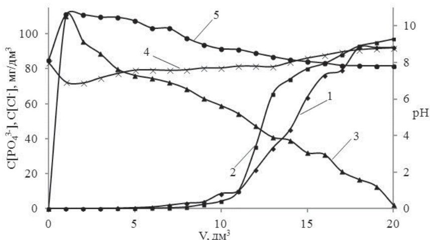
Рис. 1. Залежність вихідної концентрації фосфатів (1; 2), хлоридів (3), pH-середовища (4; 5) від об'єму пропущеного розчину фосфату натрію ( C(\text{PO}_4^{3-}) = 92 мг/дм 3 (1; 3; 4), 97 мг/дм 3 (2; 5); L = 1,5 мг-екв/дм 3 ; pH = 8,00) через аніоніт АВ-17-8 ( V_i = 20 см 3 ) в Cl - (1; 3; 4) та OH - (2; 5) формі. (ОДЄ 1 пр = 290 мг-екв/дм 3 , ПОДЄ 1 = 1888 мг-екв/дм 3 ; ОДЄ 2 пр = 995 мг-екв/дм 3 , ПОДЄ 2 = 1950 мг-екв/дм 3 )
