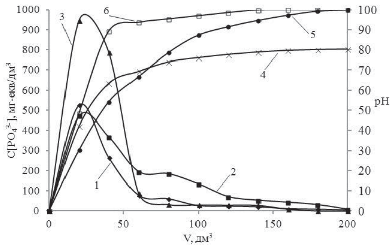
Рис. 7. Залежність вихідної концентрації фосфатів (1; 2; 3) та ступеню їх десорбції (4; 5; 6) від пропущеного об'єму розчину хлориду натрію концентрацією 10% (1; 4) та 15% (2; 5), та розчину хлориду амонію концентрацією 10% (3; 6) через аніоніт АВ-17-8 в PO_4^{3-} формі ( V_i = 20 \text{ см}^3 )
