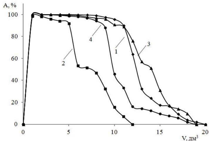
Рис. 5. Залежність ступеню вилучення фосфатів на аніоніті АВ-17-8 ( V_i = 20 \text{ см}^3 ) в \text{OH}^- (1; 2) та \text{Cl}^- (3; 4) формі з модельних розчинів ( \text{C}(\text{PO}_4^{3-}) , \text{мг/дм}^3 : 97 (1), 92 (3)) та водопровідної води ( \text{C}(\text{PO}_4^{3-}) , \text{мг/дм}^3 : 83 (2), 105 (4)) від об'єму профільтрованого розчину
