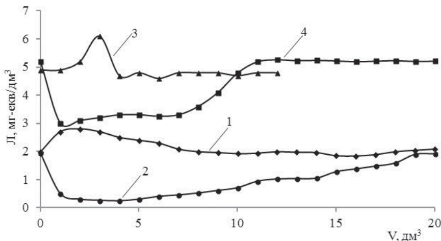
Рис. 6. Зміна лужності модельного розчину ( \text{C}(\text{PO}_4^{3-}) , \text{мг/дм}^3 : 97 (1), 92 (2)) та водопровідної води ( \text{C}(\text{PO}_4^{3-}) , \text{мг/дм}^3 : 83 (3), 105 (4)) в залежності від пропущеного об'єму через аніоніт АВ-17-8 ( V_i = 20 \text{ см}^3 ) в \text{OH}^- (1; 3) та \text{Cl}^- (2; 4) формі
