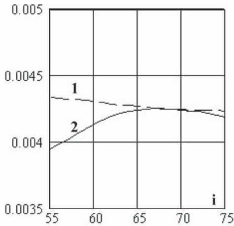
Рис. 5. Порівняння розрахованих за (18), крива 1 та вимірених концентрацій \text{Ca}^{2+} , крива 2, \text{М/дм}^3 .
