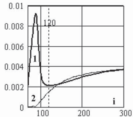
Рис. 14. Залежність концентрації твердого CaCO_3 від номеру вимірювання i . Крива 1 - розрахунок за (33), 2 - за (20).
