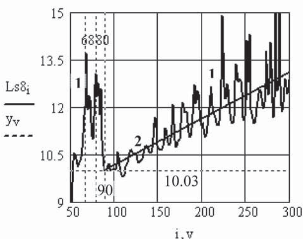
Рис. 9. Залежності (29), крива 1 та (30), лінія 2, від номеру виміру. Цифри 68, 80 та 90 вказують на значення номерів вимірів, цифра 10.3 – значення функції (29) в точці i = 90 .
