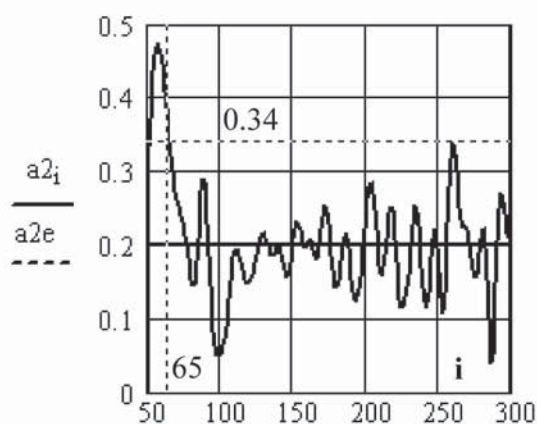
Рис. 2. Поточні значення параметра десорбції a_2 залежно від номера виміру i . Середнє від a_2 на проміжку 50 < i < 300 в просторі індексів i рівне 0.2, а в часі 0.2/27 = 7.41 \cdot 10^{-3} \text{ c}^{-1} .
