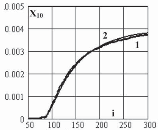
Рис. 7. Концентрація скристалізованого \text{CaCO}_3 , розрахована за (20), крива 1 та інтегруванням (25), крива 2.
