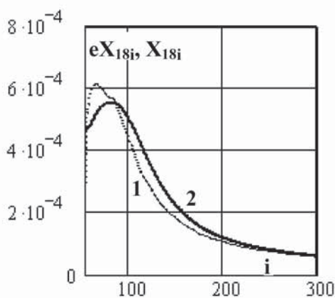
Рис. 3. Залежність концентрації, \text{М}/\text{дм}^3 , комплексів \text{CaHCO}_3^+ від номеру виміру i . Крива 1-рівноважне значення; крива 2 - розраховане за (16), \Delta i = 27\text{с} .
