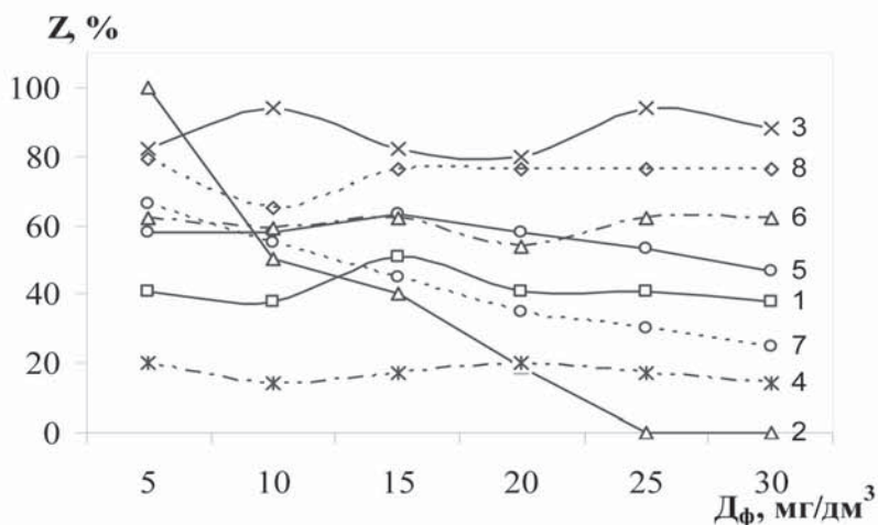
Рис.1. Влияние дозы флокулянтов ПОПМЭА (1-3) и ПОПДМАХ (4-8) на степень очистки воды от урана при дозе коагулянтов: РИКС-А0 0,0 \text{ мг/дм}^3 (1,4) (pH=8,0); 10 \text{ мг/дм}^3 , pH=8 (2,7); pH=4,0 (5); pH=6,0 (6); 20 \text{ мг/дм}^3 ; pH=8 (3); Полвак-68 10 \text{ мг/дм}^3 , pH=8,0 (8).
