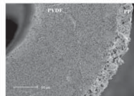
Рис. 6. Композитная ультрафильтрационная полволоконная мембрана.
